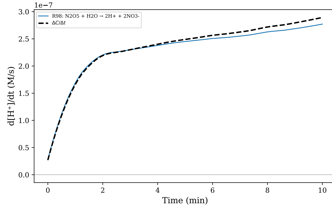
(d) H + [final=140.85 μM]
